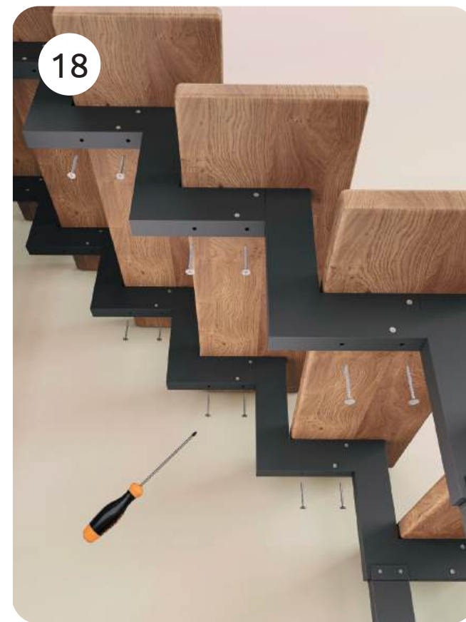
18. Фиксируем ступени: • треугольные ступени • прямые
