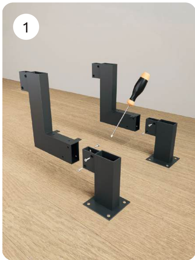
1. Сборка нижнего модуля.
