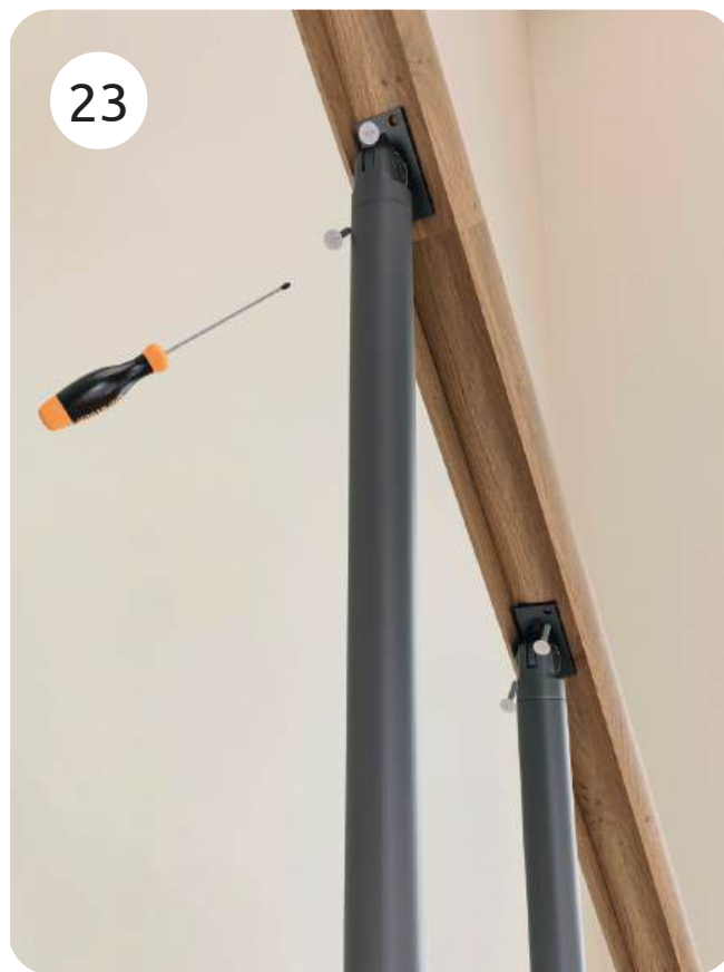
23. Фиксируем поручень к опорам саморезами.
