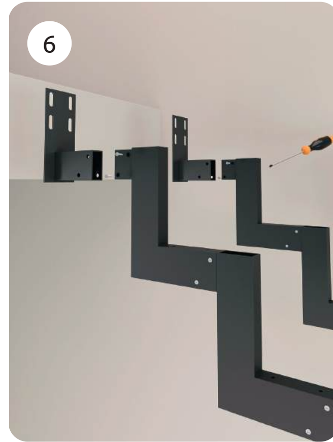
6. Сборка верхнего модуля.
